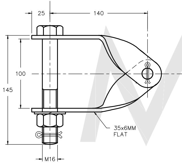
CROSSARM STRAP
